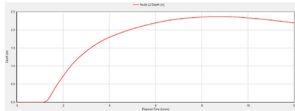
Figura 4: Nivel alcanzado en el espacio de laminación II, para la lluvia de 81mm
